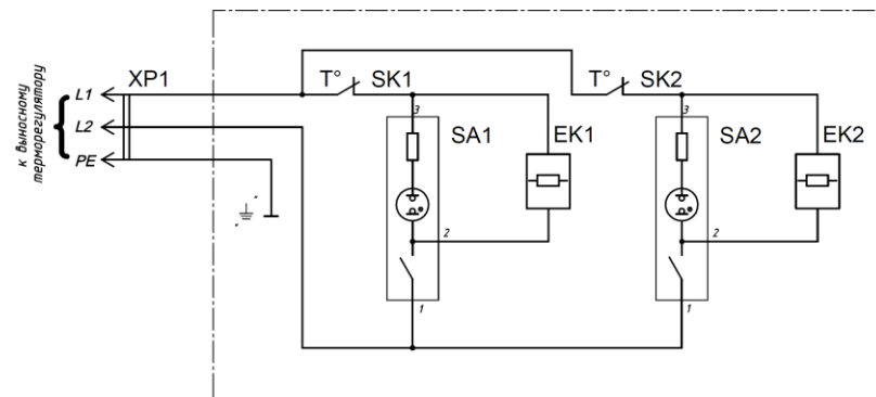
Схема электрическая принципиальная
