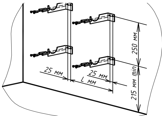
Рисунок 2 – Порядок установки кронштейнов
